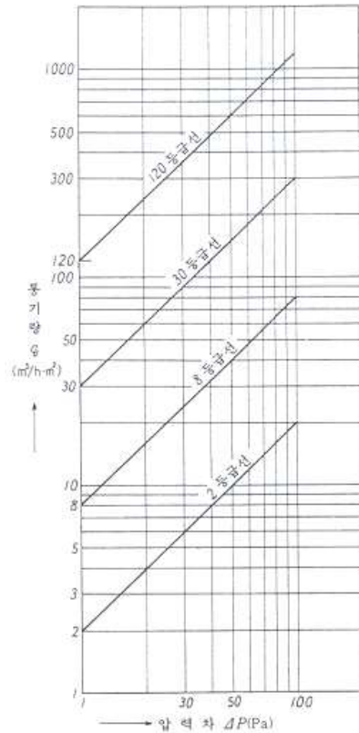
[그림 8] 기밀성 등급 선
