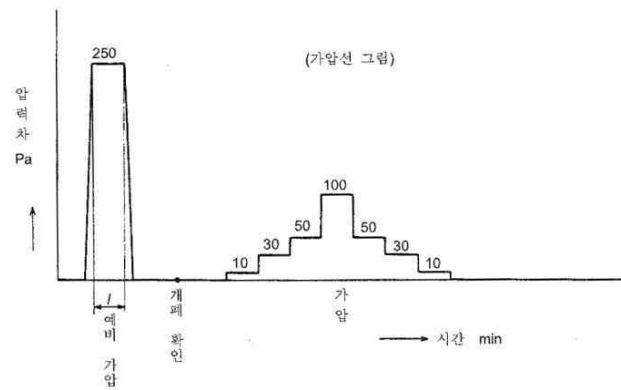
[그림 7] 기밀성 시험 순서
