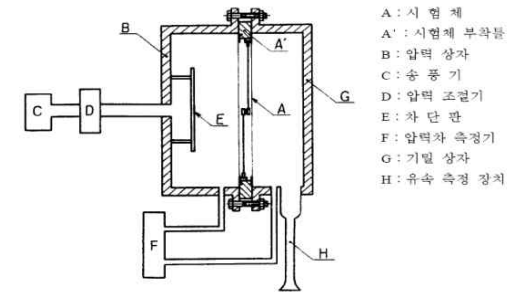
[그림 6] 기밀성 시험장치
